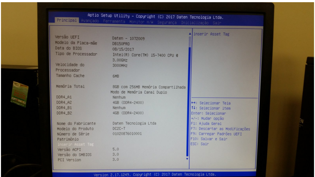
Foto 10: Desktop - BIOS
